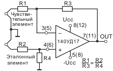
Высокостабильный усилитель терморезистора
