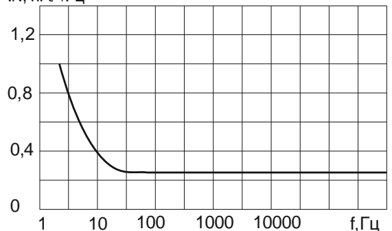
Рис.10 Зависимость спектральной плотности тока шума от частоты
