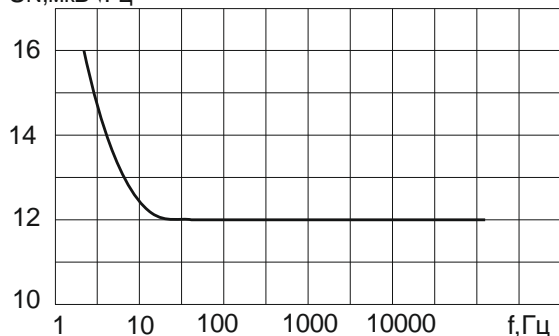
Рис.9 Зависимость спектральной плотности напряжения шума от частоты
