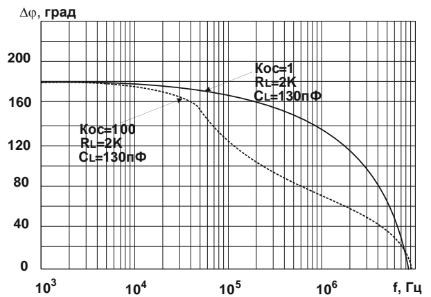
Рис.6 Зависимость фазо-частотных характеристик для различных коэффициентов усиления с ОС
