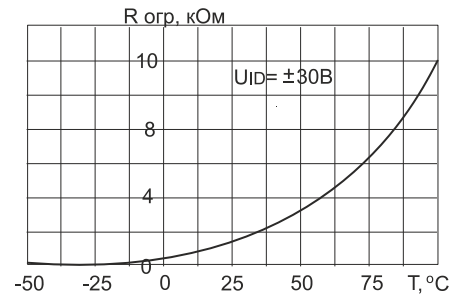
Рис.4 Зависимость минимально-допустимого входного ограничительного сопротивления от температуры окружающей среды
