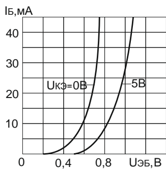
Входные характеристики
